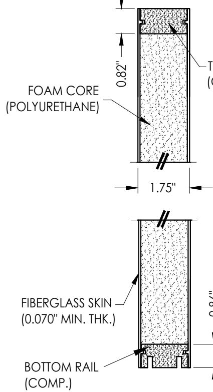
SECTION D-D
